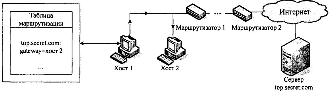
Рисунок 8. Схема реализации атаки "Навязывание ложного маршрута" (внутрисегментное) с использованием протокола ICMP с целью нарушения связи
